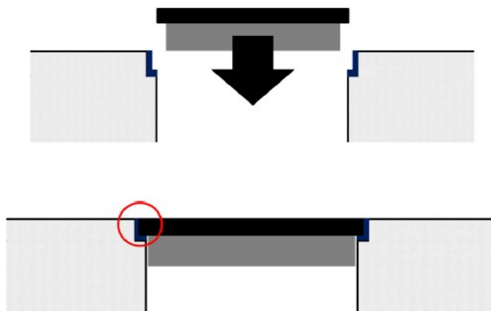
Joint silicone et montage en affleurement
